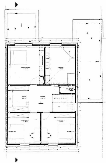
00_vloerpl.1 - NT
