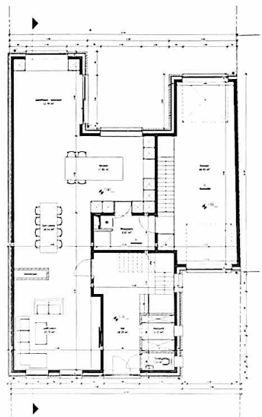
00_gr.vloers - NT
